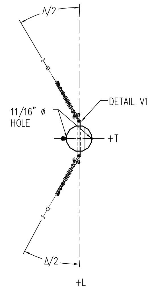
SECTION D-D (N.T.S.)
