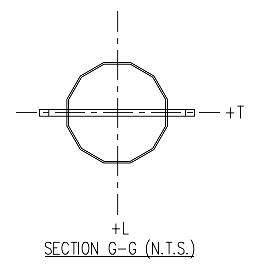
SECTION G-G (N.T.S.) TWO WAY ONE HOLE THROUGH VANG - VERTICAL (N.T.S.)
