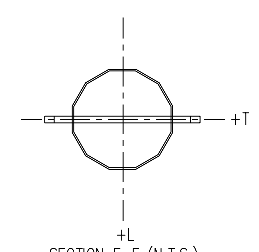
SECTION F-F (N.T.S.) TWO WAY ONE HOLE THROUGH VANE - VERTICAL (N.T.S.)
