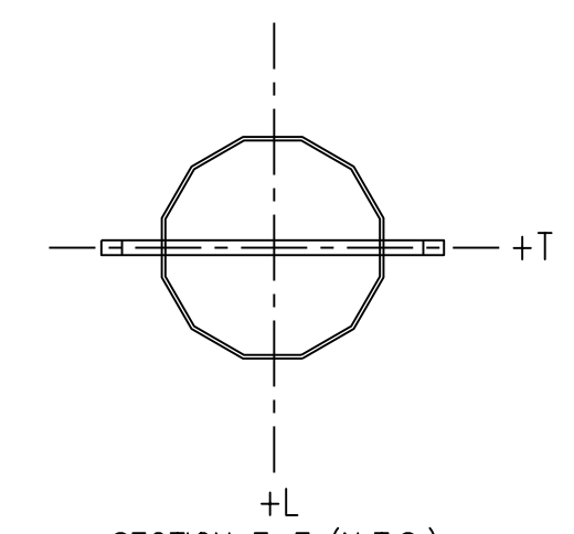
SECTION F-F (N.T.S.)
