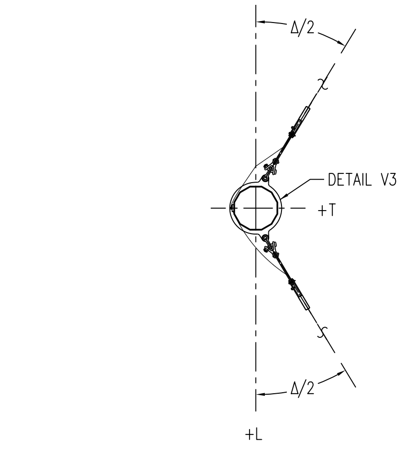
SECTION A-A (N.T.S.) OHGW ATTACHMENT 7/9" ALUMOWELD
