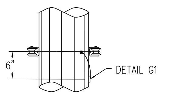
SECTION G-G (N.T.S.)
