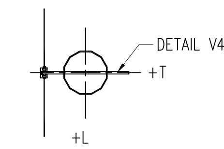
SECTION A-A (N.T.S.) OHGW ATTACHMENT 7#9 ALUMOWELD
