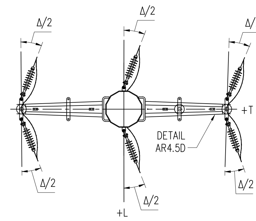
SECTION C-C (N.T.S.) DISTRIBUTION ATTACHMENT 795 KCMIL 37/0 STRAND "ARBUTUS" AAC
