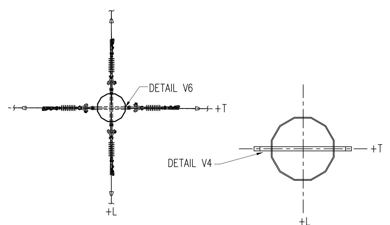
SECTION G-G (N.T.S.) NEUTRAL ATTACHMENT 336.4 KCMIL 18/1 STRAND "MERLIN" ACSR SECTION I-I (N.T.S.) TWO WAY ONE HOLE THROUGH VANG - VERTICAL (N.T.S.)
