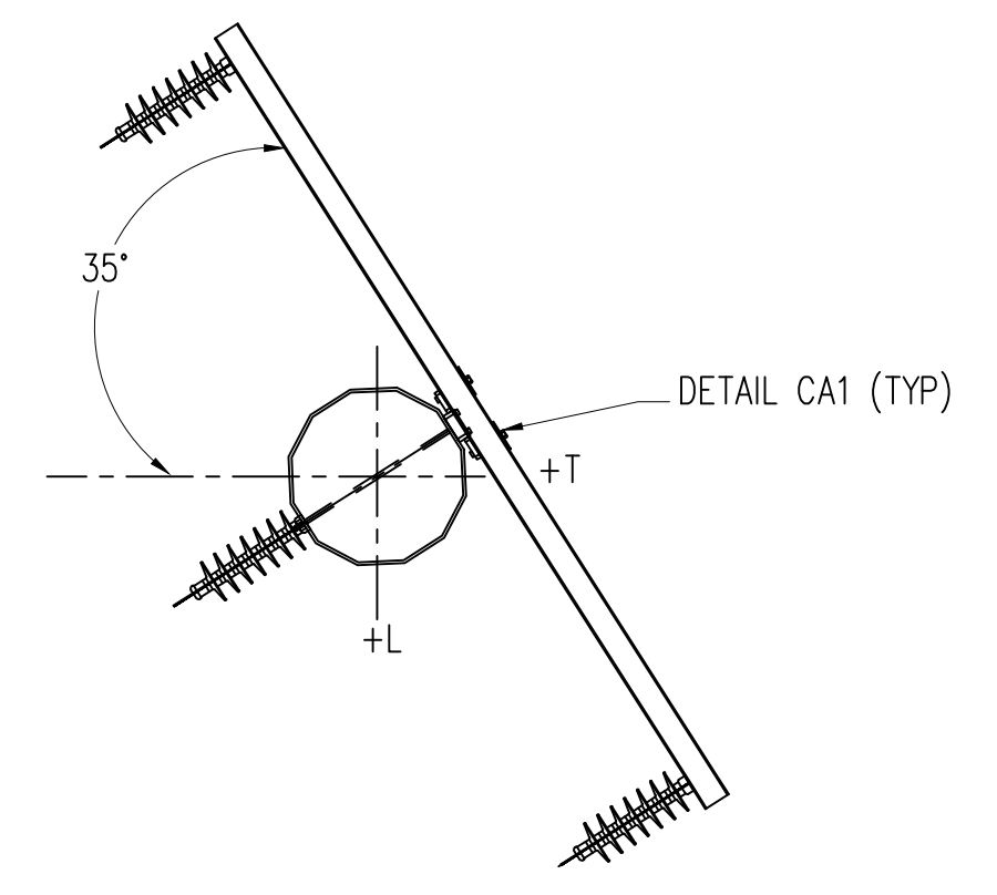
SECTION D-D (N.T.S.) DISTRIBUTION ATTACHMENT 795 KCMIL AAC "ARBUTUS"
