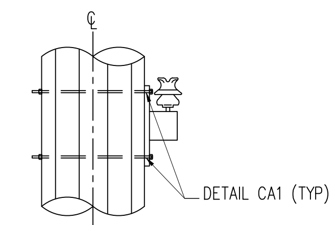
SECTION K-K (N.T.S.) DISTRIBUTION ATTACHMENT 795 KCMIL AAC "ARBUTUS"
